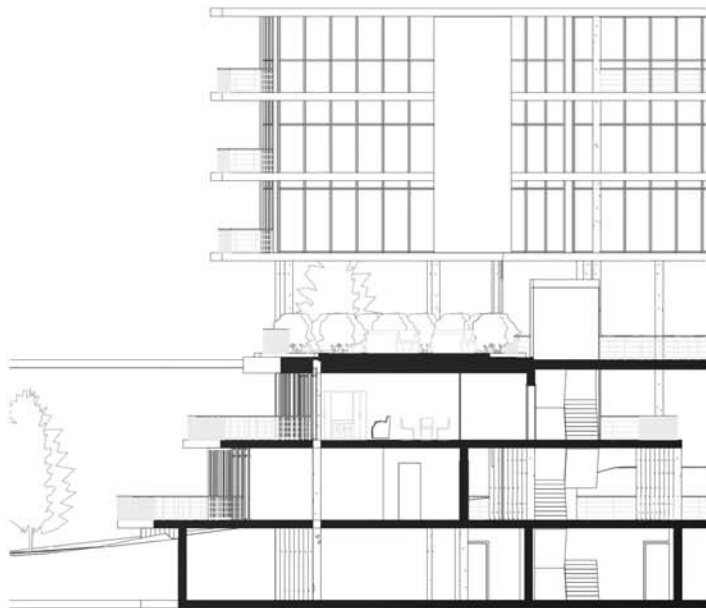
Sezione ballatoio Scala 1:200
