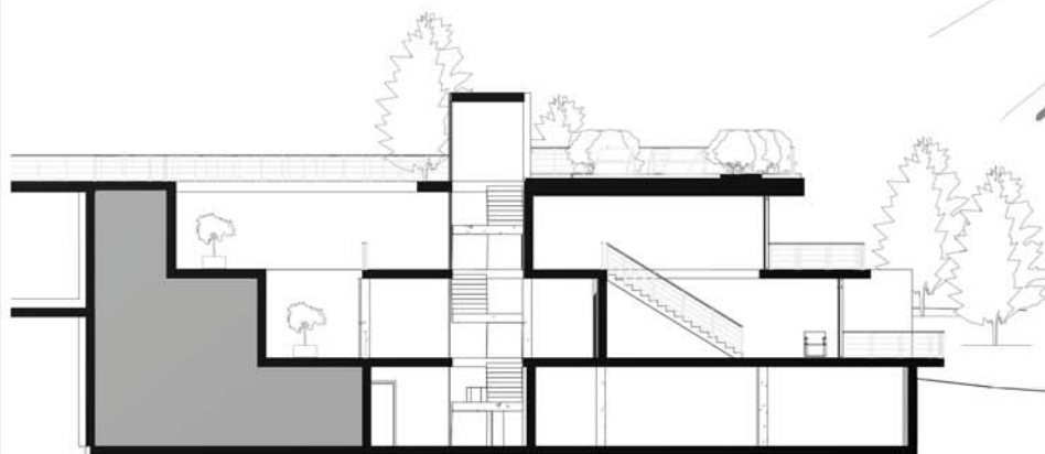
Sezione duplex ballatoio Scala 1:200
